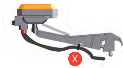
Anschlussleitung nicht mit Kabelbindern fixieren.
