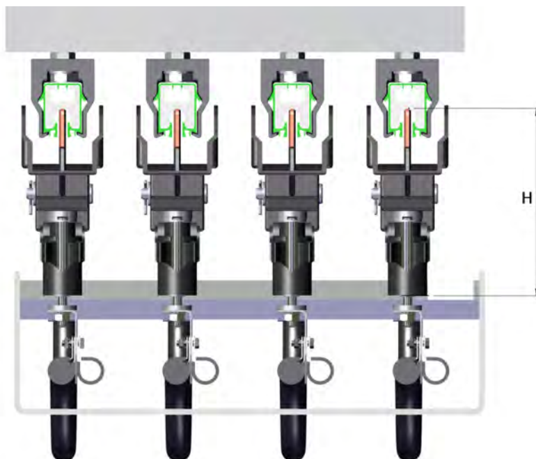
Stromabnehmer der Typenreihe UST 200/35 und UDST 400/35
