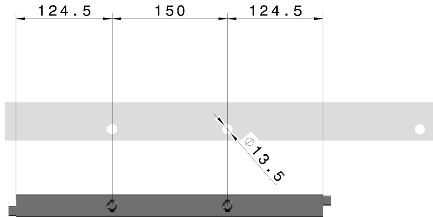
Lochbild Einspeisung
