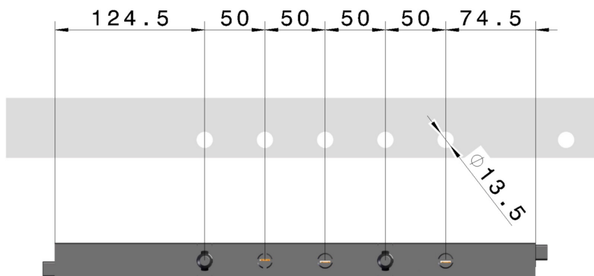
Lochbild Auffahrrampe
