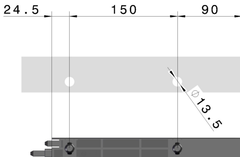
Lochbild Auffahrrampe
